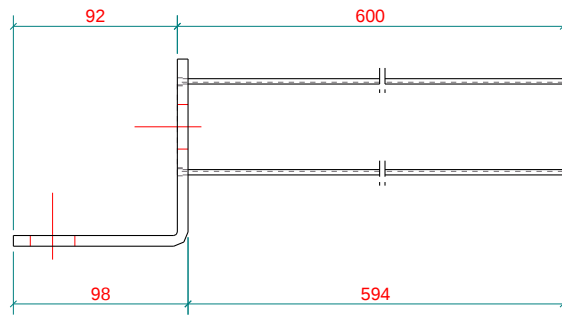
SECTION B - B 1:3
