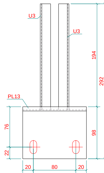
SECTION A - A 1:3
