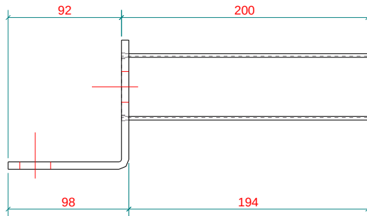
SECTION B - B 1:3
