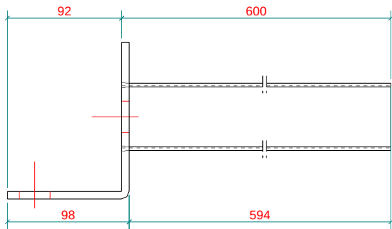
SECTION B - B 1:3
