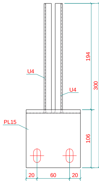
SECTION A - A 1:3
