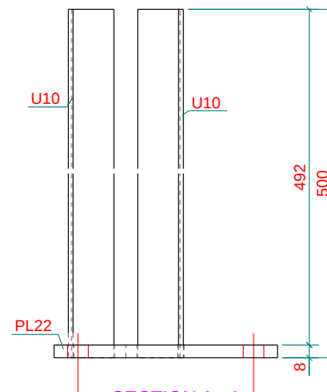
SECTION A - A 1:3
